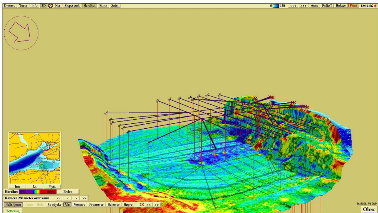
Figur 7. Bunnkartlegging 3D visning havbunn WASSAP multistråledata (Backscatter). Sett fra sør mot nord Olex.
