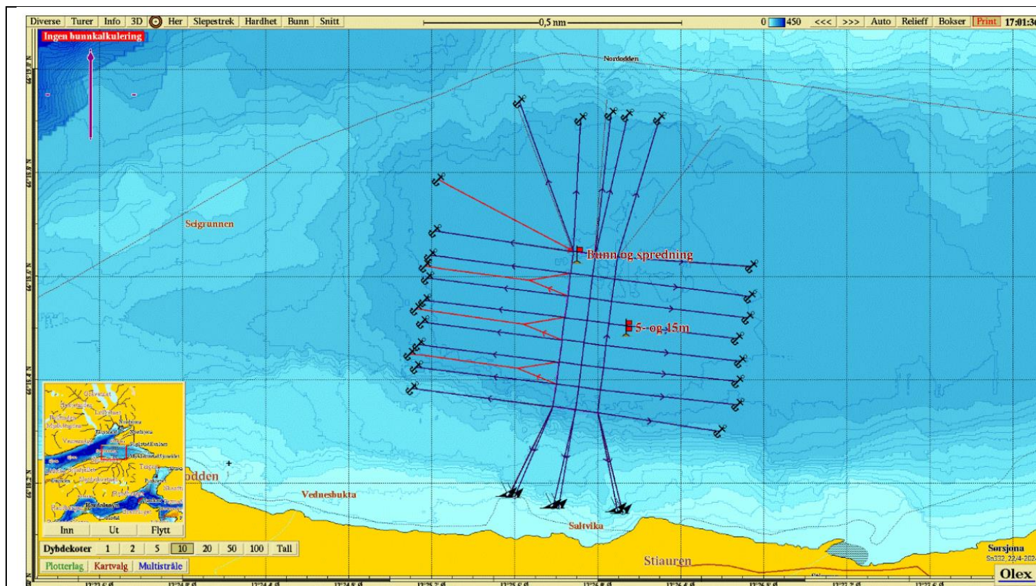
Figur 3.1.1. Plassering av strømrigger relativt til anleggsrammen.
