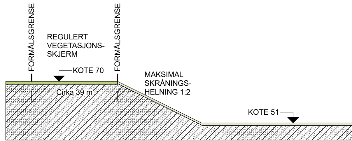
SNITT A
