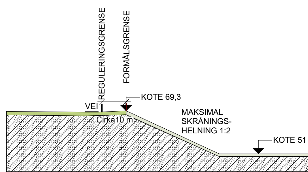
SNITT B
