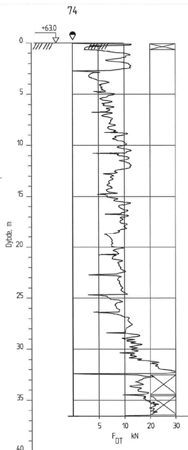
Figur 3-4: Sondering utført ca. 80 m sørøst for planområdet. Utklipt fra [1].
